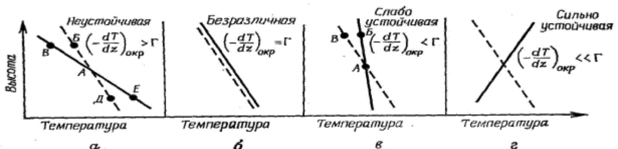
Рис.2.1 – Градиент температуры и устойчивость атмосферы
