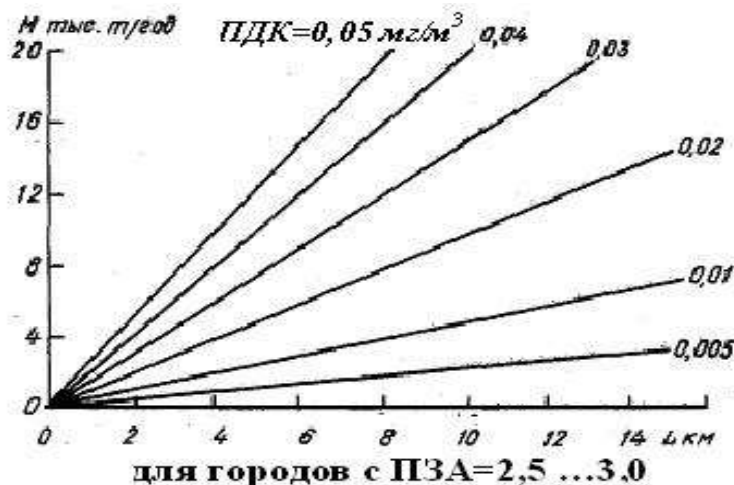
Рис. 10.1 – Зависимость между суммарными выбросами M , характерным размером города L и средней концентрацией примеси ПДК с.с.
