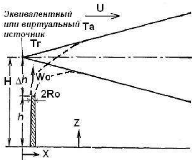
Рис.1.2 – Виртуальный источник с эффективной высотой H .
